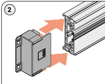
2- Modülü, FL-I busbarın son ucuna tırnakların içine oturacak şekilde takınız.
