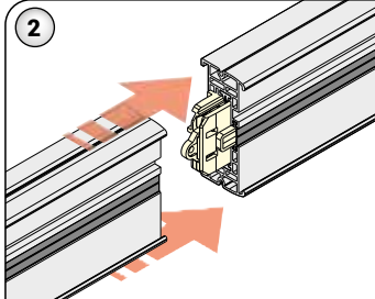
2- Ekleniecek diğer FL-I Busbarı, aynı şekilde iletkenler ek elemanı kontaktlarının arasına girecek şekilde yerleştiriniz ve tam oturduğundan emin olun.
