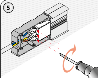
5- Besleme kablosu uçlarını (L/N/PE) ilgili klemenslere sabitleyiniz ve kablo kelepçesini sıkınız.
