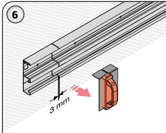
6- FLD ek noktalarında 3mm boşluk bırakıldığından, el masterı yardımıyla kontrol ederek, emin olunuz.
