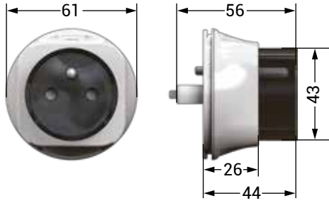
Fransız Standartı Topraklı Priz (UPS)
