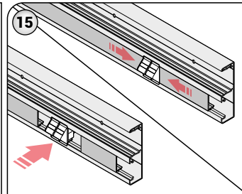
15- FLD Datalı Busbar Data&Telefon priz kaidesini, kanal üzerine yerleştiriniz. FLD Datalı Busbar kapağını iterek priz kaidesini sıkıştırınız.
