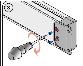
3- Modül takıldıktan sonra şekilde görüldüğü gibi FL-I Busbara vidalayarak sabitleyiniz.
