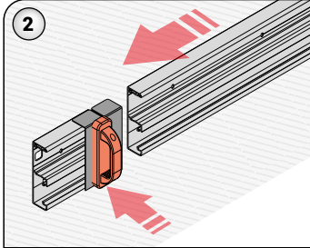
2- FLD ek noktasında 3mm boşluk bırakınız. Bunun için, ürün ile birlikte verilen el masterını kullanınız.
