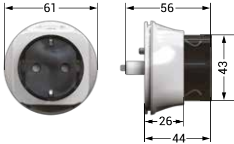
Alman Standartı Topraklı Priz (Şebeke)
