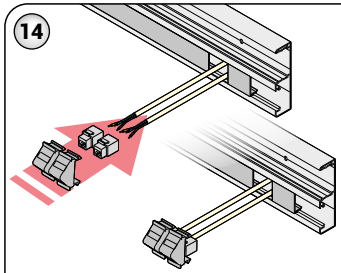
14- Kabloların, RJ45 data prizlerine, uzman bir eleman tarafından çekilmesini sağlayınız ve kabloları çekilen RJ45 data prizlerini; FLD Datalı Busbar Data&Telefon priz kaidesine yerleştiriniz.
