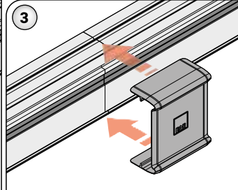
3- Ek elemanı kapağı, busbarların ek noktasını ortalamak ve tırnakları gövde yarığı içine girecek şekilde takınız.
