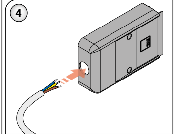
4- Besleme kablosunu, uçlarını soyarak delikten geçirin.
