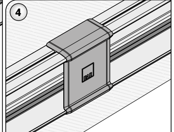
4- Ek Elemanı kapağının tam olarak yerine oturduğundan emin olun ve montajı sonlandırınız.
