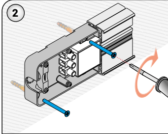
2- FL-I Besleme Modülünün kapağını çıkartınız ve 2 adet M6 dübel ve vida ile duvara sabitleyiniz.
