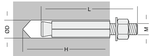
Gömlekli Dübel
